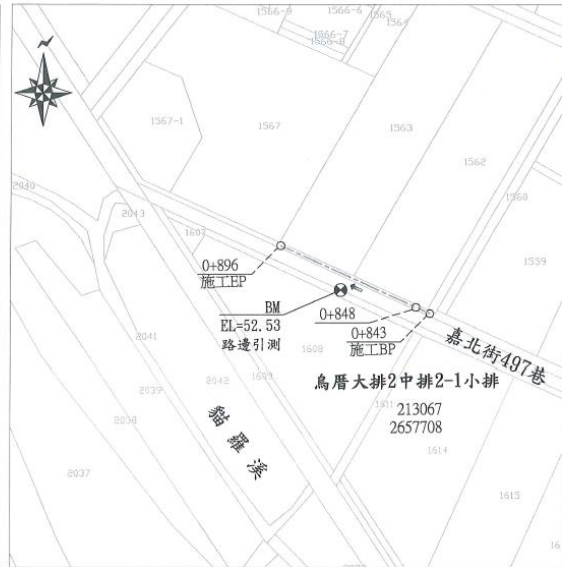
烏厝大排2中排2-1小排 施工位置圖 芬園鄉嘉北段 S=1/1000
