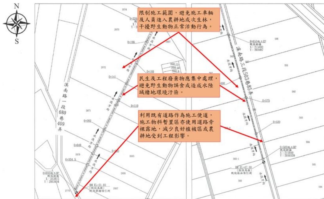
溪渠排水20-2小排 烏日區溪南西段 平面位置圖 S=1/1000 (座標系統 97TM2)
