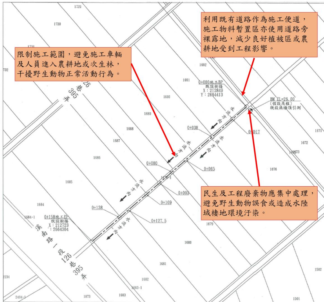
溪渠排水東園1圳支線2分線3-2小給 烏日區溪南西段 平面位置圖 S=1/1000 (座標系統 97TM2)
