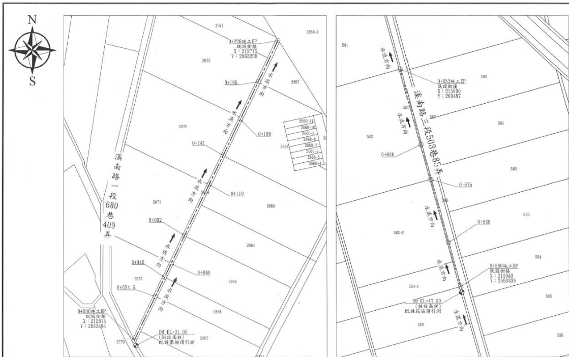
溪墘排水20-2小排 烏日區溪南西段 平面位置圖 S=1/1000 (座標系統 97TM2)
